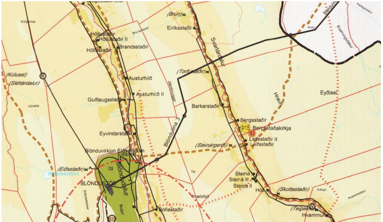
Mynd 2. Hluti uppdráttar úr Aðalskipulagi Húnavatnshrepps 2010 - 2022. Svört heil lína sýnir fyrirhugaða legu Blöndulínu 3 í gildandi aðalskipulagi.
